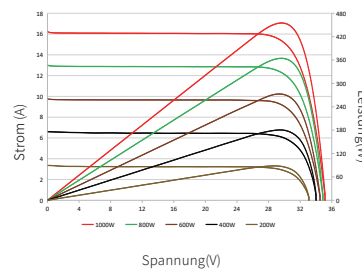
Strom-Spannungs- und Leistungs-Spannungs-Diagramme(445W)
